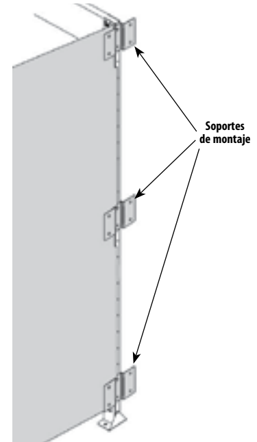
Panel posterior para estantería de almacenamiento de acero
