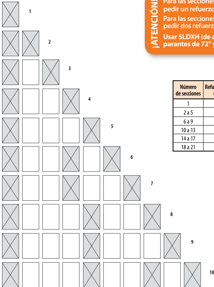
Número de refuerzos cruzados necesarios para tramos de almacenamiento en acero
